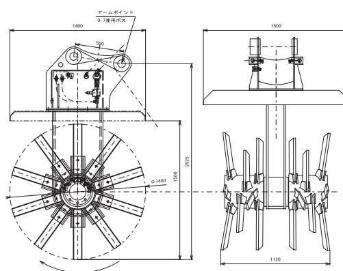
寸法図
