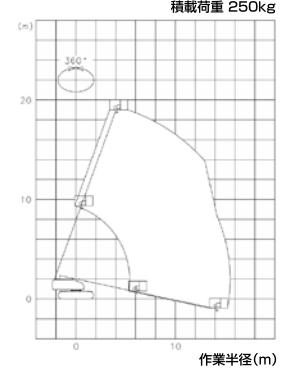
■作業範囲図
