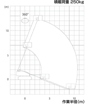
■作業範囲図
