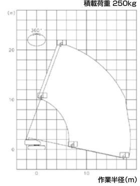
■作業範囲図
