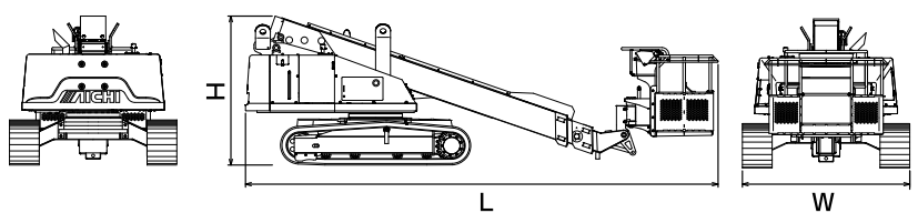
■車両寸法図
