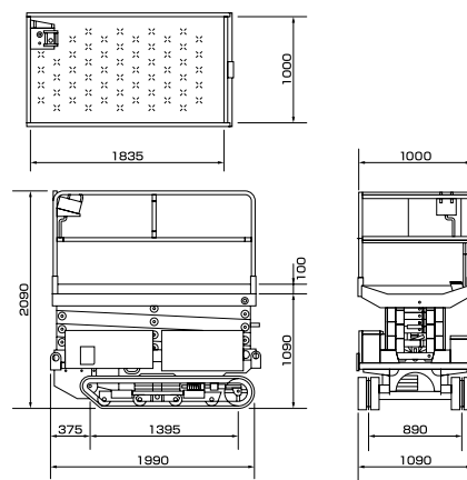
■車両寸法図
