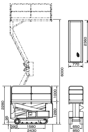
■車両寸法図
