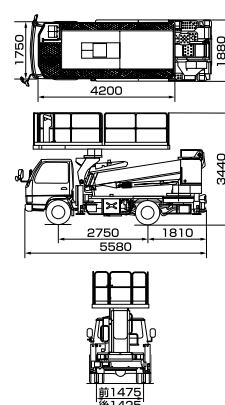
■車両寸法図
