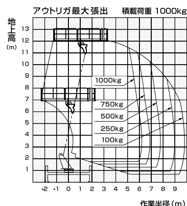
■作業範囲図
