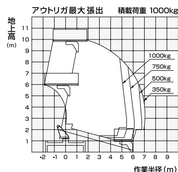
■作業範囲図
