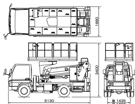
■車両寸法図
