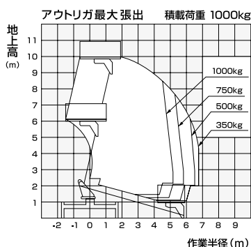
■作業範囲図
