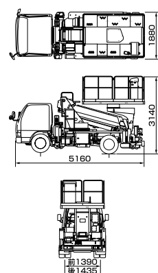
■車両寸法図
