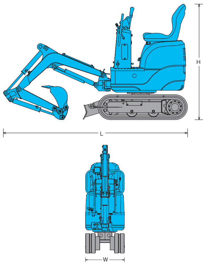
寸法図
