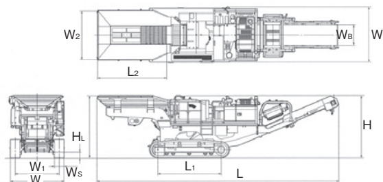
寸法図
