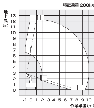
■作業範囲図
