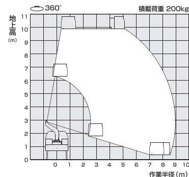
■作業範囲図
