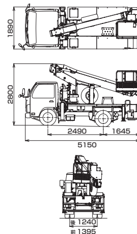
■車両寸法図
