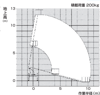
■作業範囲図
