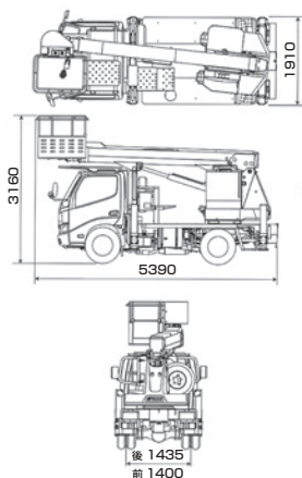
■車両寸法図
