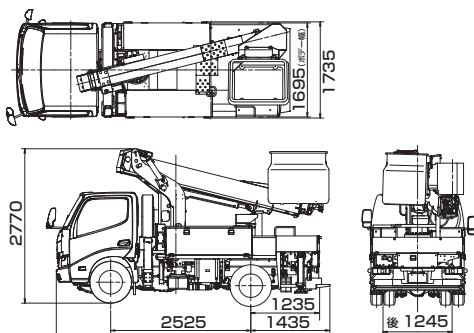
■車両寸法図
