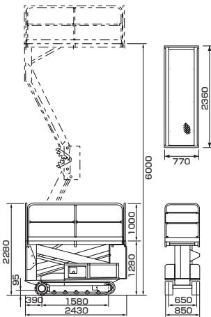
■車両寸法図
