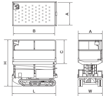
■車両寸法図
