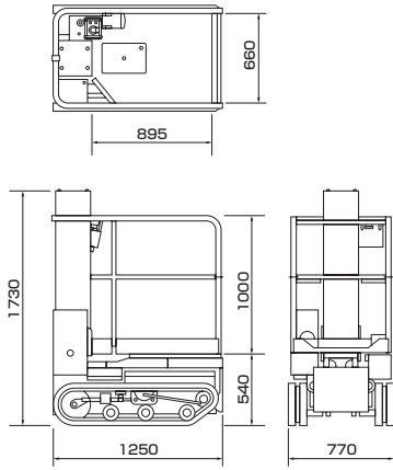
■車両寸法図
