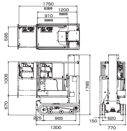
■車両寸法図
