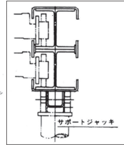
ガイドポスト断面図
