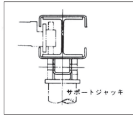
ガイドポスト断面図
