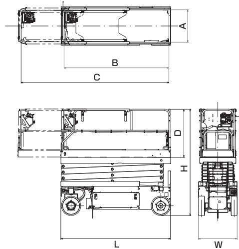
■車両寸法図
