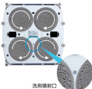
洗剤噴射口
