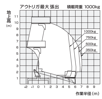
作業範囲図
