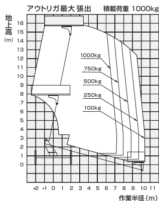
作業範囲図
