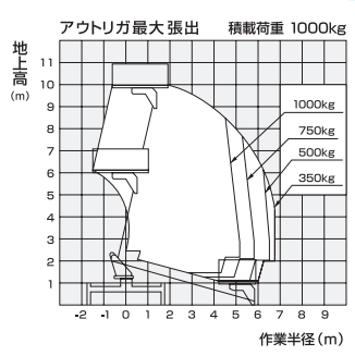
作業範囲図
