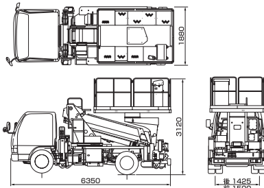
車両寸法図
