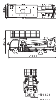
車両寸法図
