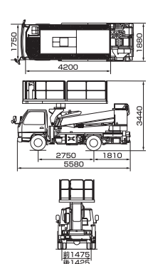
車両寸法図
