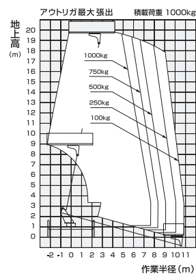
作業範囲図
