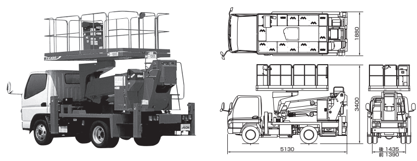
車両寸法図
