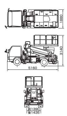
車両寸法図
