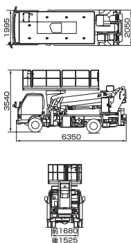
車両寸法図
