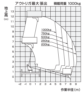
作業範囲図
