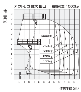
作業範囲図
