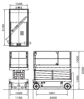
車両寸法図
