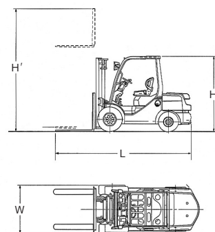
寸法図
