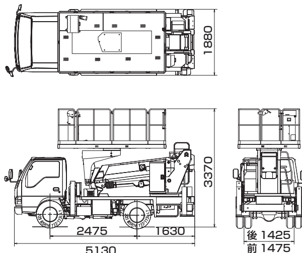
■車両寸法図
