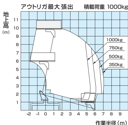
■作業範囲図
