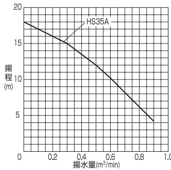
■性能曲線
