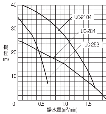
■性能曲線
