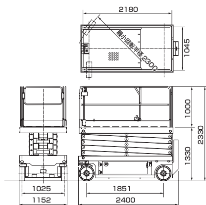
■車両寸法図
