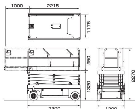
■車両寸法図
