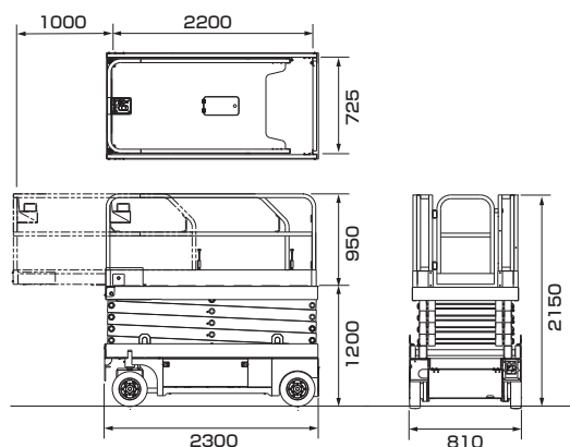
■車両寸法図
