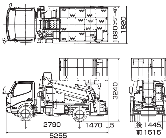
■車両寸法図
