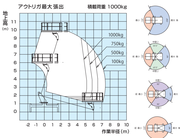
■作業範囲図
