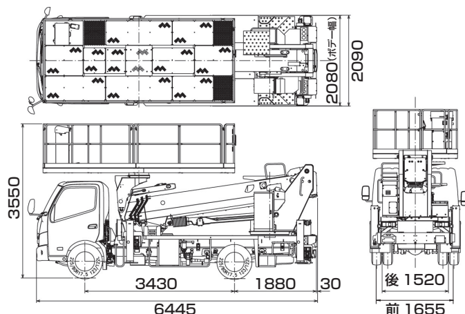
■車両寸法図
