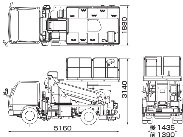
■車両寸法図
