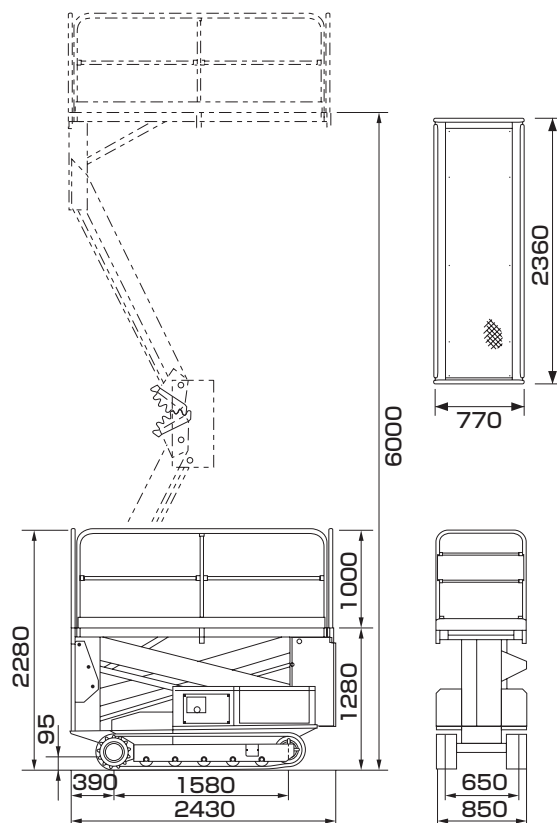
■車両寸法図
