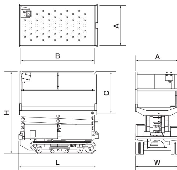
■車両寸法図
