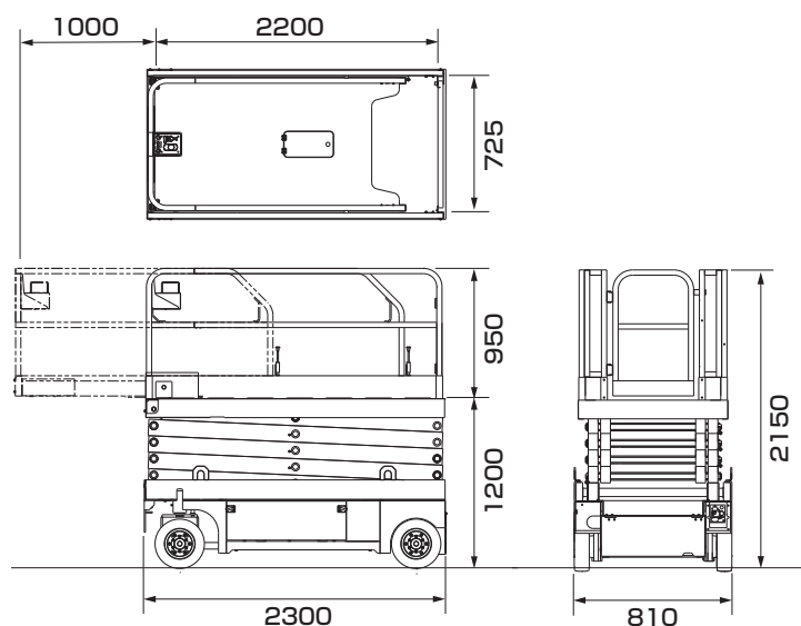
■車両寸法図
