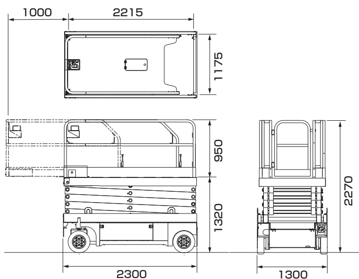
■車両寸法図
