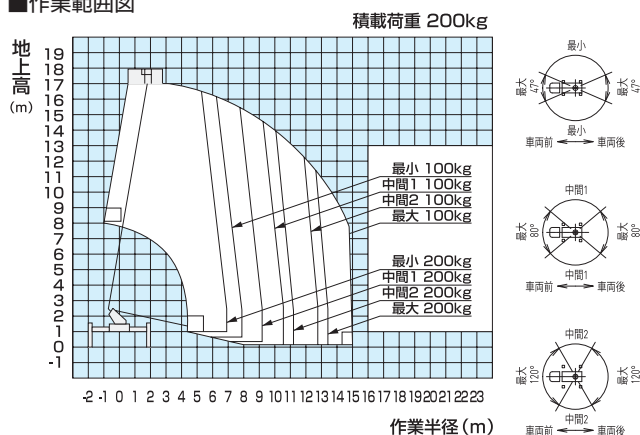
■作業範囲図
