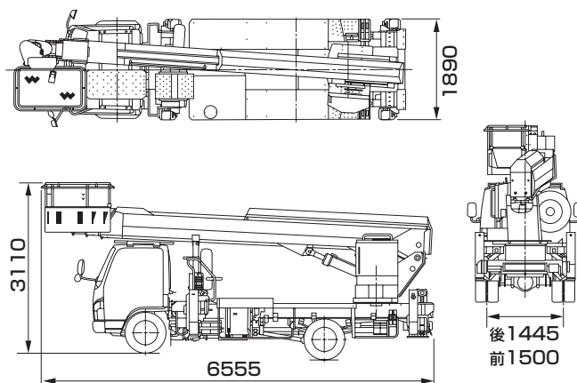
■車両寸法図
